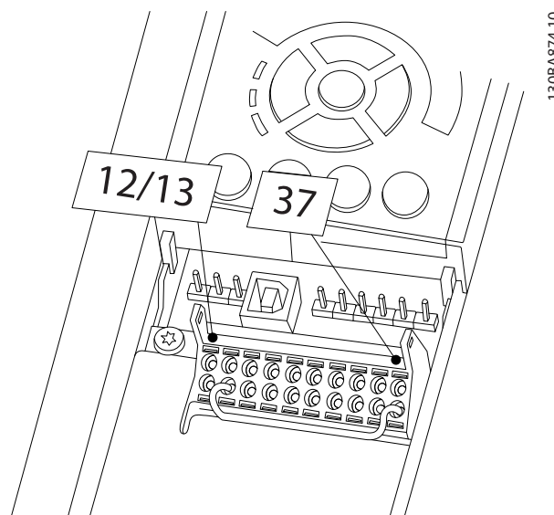
Рисунок 2.20 Соедините перемычкой клемму 12/13 (24 В) и клемму 37.
