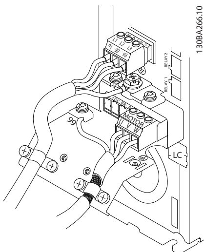
Рисунок 2.10 Проводка двигателя, силовых кабелей и заземления для типоразмеров A
