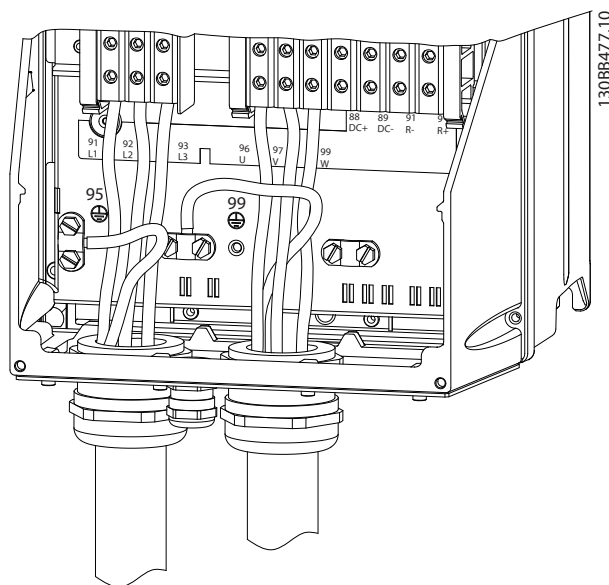
Рисунок 2.12 Проводка двигателя, силовых кабелей и заземления для типоразмеров B и выше с использованием кабелепровода
