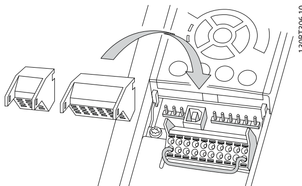
Рисунок 2.17 Отключение клемм управления
