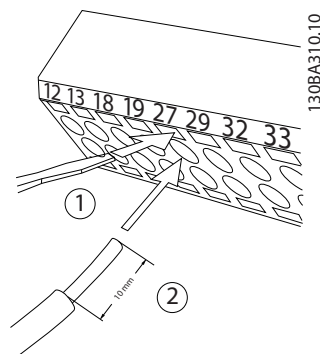
Рисунок 2.18 Подключение элементов управления
