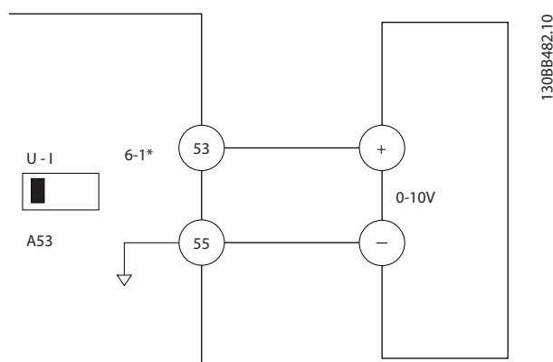
Рисунок 5.1 Пример подключения к внешнему устройству с управляющим сигналом 0–10 В
